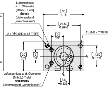
ANSICHT: A-A
