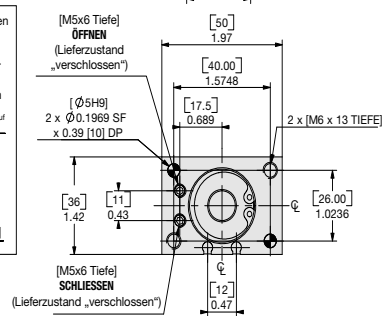
ANSICHT: A-A
