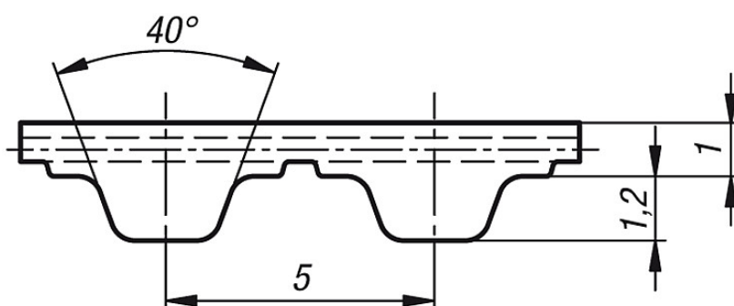
Profil T5
