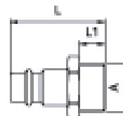
Nippel Außengewinde
