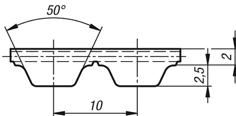
Profil AT10
