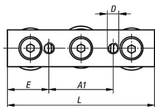
Loslager Massivausführung
