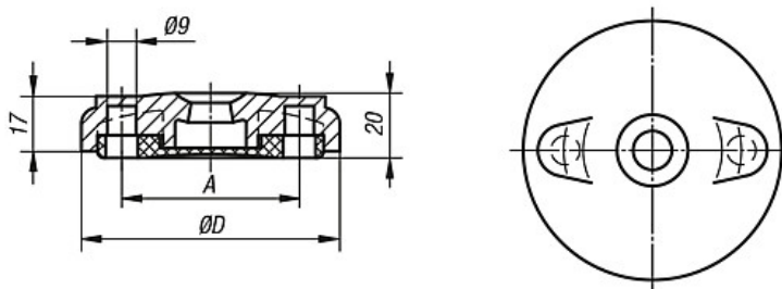
Form D mit Anschraubbohrung (geschlossen) mit Anti-Slip-Platte
