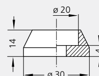
Edelstahl-Abschlusscheibe für Ø 20 Stainless steel cover plate for Ø 20
