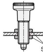
Rastbolzen GN 613
