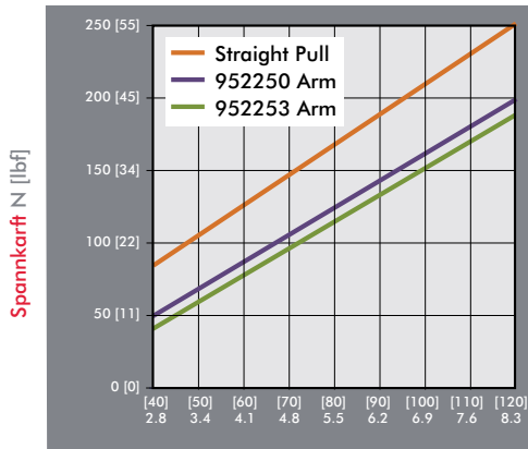
Serie 9522 Kolbenkraft
