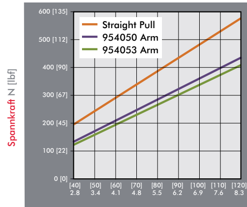
Serie 9530 Kolbenkraft
