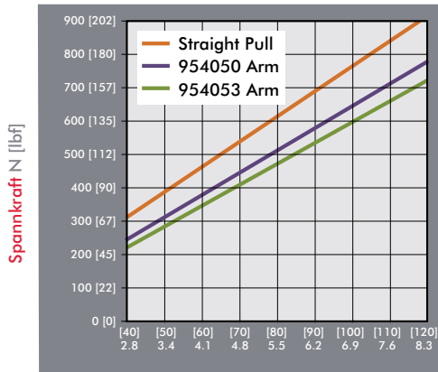
Serie 9540 Kolbenkraft
