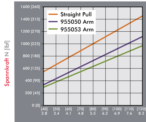
Serie 9550 Kolbenkraft
