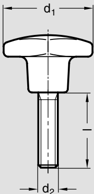
Form SK Kreuzgriff DIN 6335 Kunststoff (KU) Duroplast PF 31 LE.-Nr. 04433 Kat. 8.1. Seite 111
