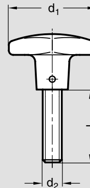
Form SG Kreuzgriff DIN 6335 Gußeisen (GG) LE.-Nr. 04301 Kat. 8.1. Seite 110
