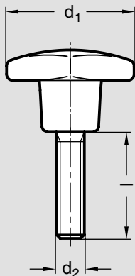
Form ST Sterngriff DIN 6335 Kunststoff (KT) Thermoplast (Polyamid PA)
