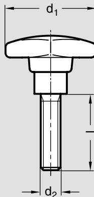
Form TE Kreuzgriff DIN 6335.2 Kunststoff Thermoplast (Polyamid) LE.-Nr. 04465 Kat. 8.1. Seite 111
