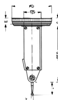
Form C nach DIN 2270
