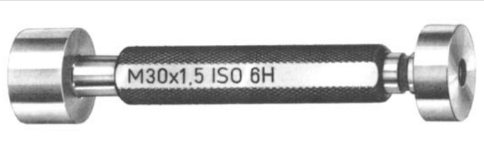
Grenzlehrdorn Nr. 101 K für den Kerndurchmesser des Mutterge- windes
