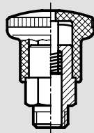
Form C (ausgerastet Knopf 30° gedreht)
