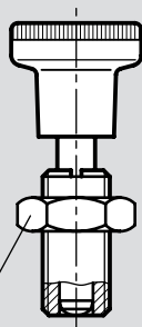
Kontermutter ISO 8675
