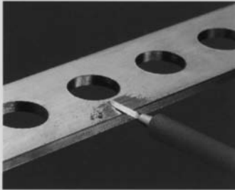
MINI-DREIKANTSCHABERER FT 1100 für feine und diffizile Arbeiten
