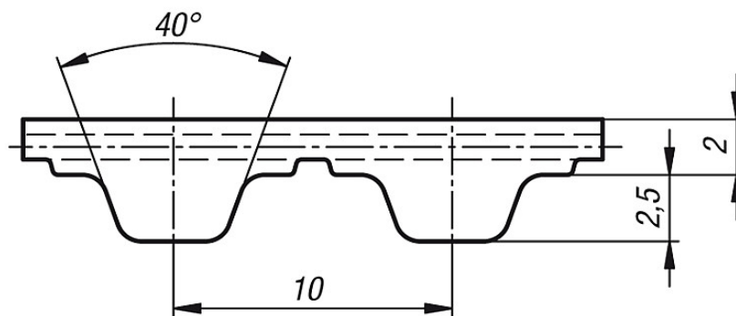
Profil T10
