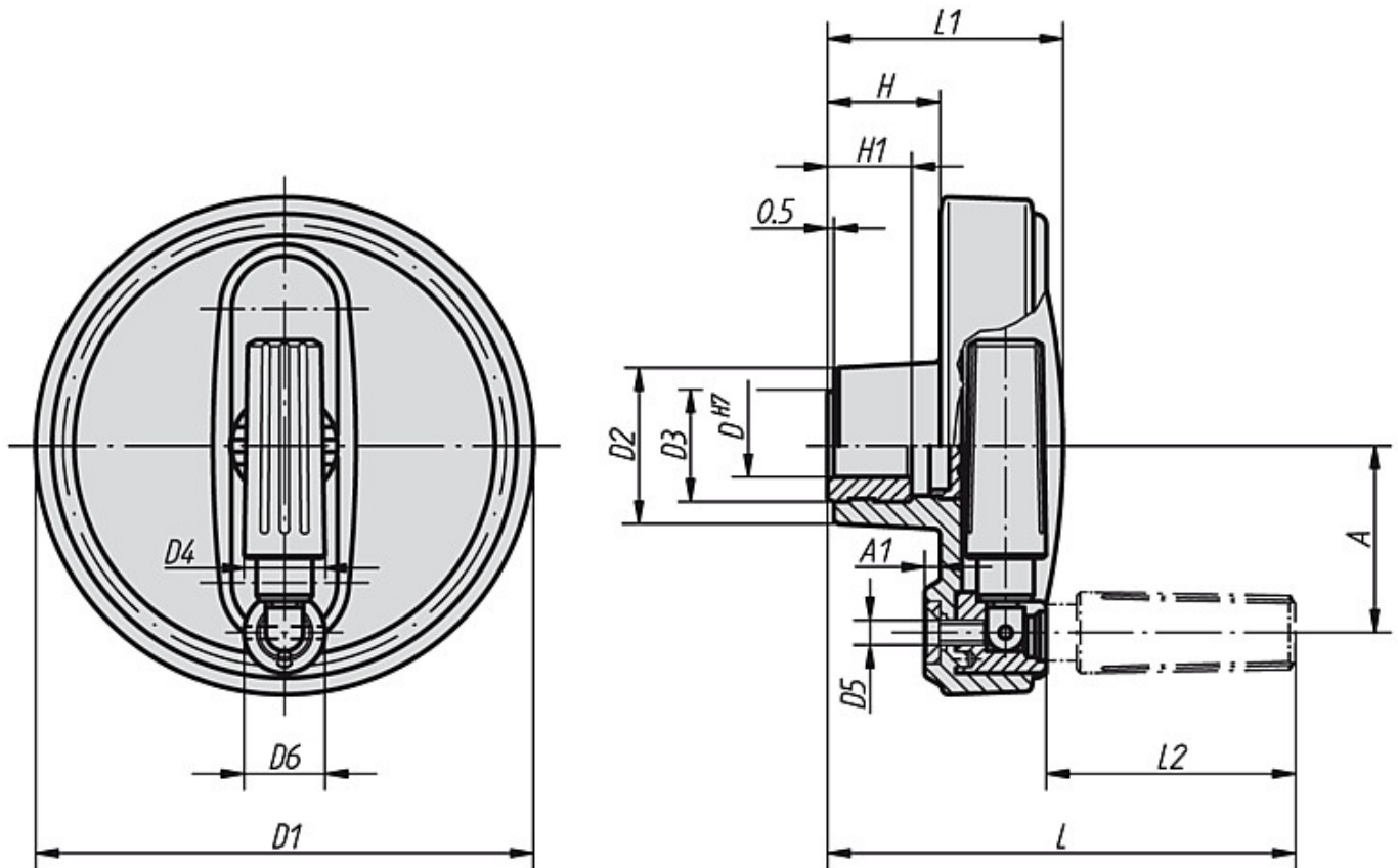
Nabennut nach DIN 6885-1
