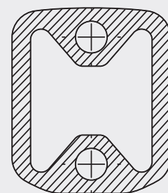
Griffquerschnitt M 1:1 Handle cross section scale 1:1
