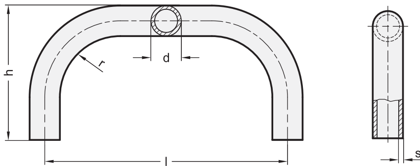
4 Form A einfach gebogen, 90°
