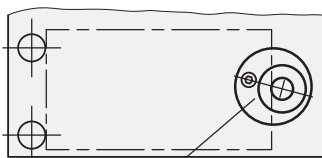
Exzenterbuchse GN 715.2
