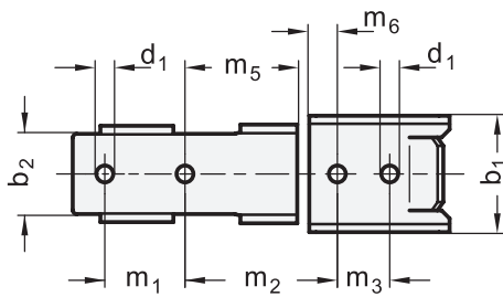
Bohrbild für b_1 = 15 / 20 / 29
