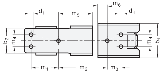
Bohrbild für b_1 = 40
