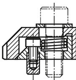
Schnitt A-A
