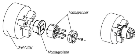
Montageplatte zum Einsetzen der Spannzange auf Drehmaschine
