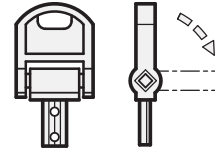
Schlüssel Form CSF (Kugelknopf)
