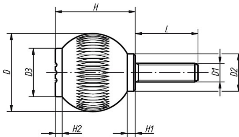
Griffkugel mit Außengewinde
