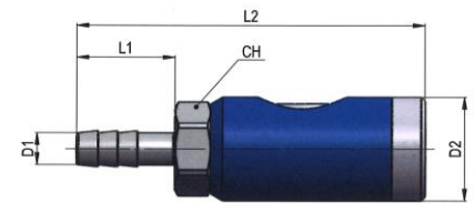
Schlauchtülle
