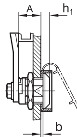
Verriegelungen GN 115
