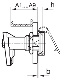
Türverriegelung GN 119
