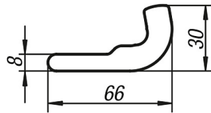
Gegenhaken Form B (anschweißbar)
