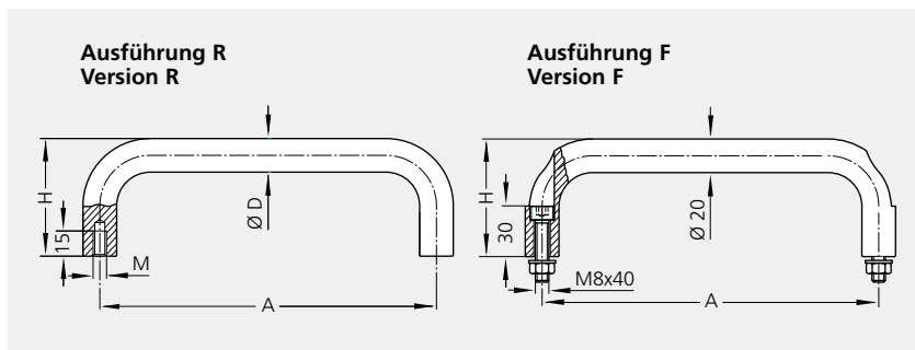
Ausführung M1-20.F (Abschlusscheibe optional) Version M1-20.F (cover plate optional)
