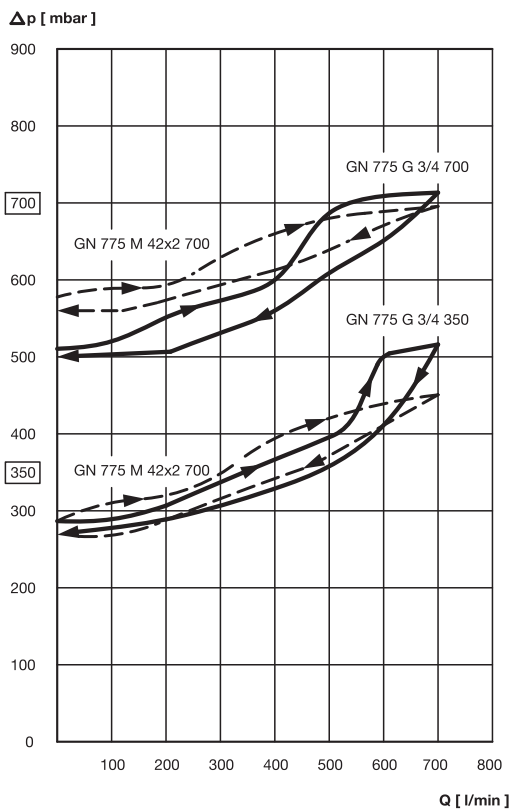
Druckverlauf \Delta p [mbar] im Behälter in Abhängigkeit vom Luftdurchsatz [l/min.] bei Ventilöffnungsdruck 350 bzw. 700 mbar.
