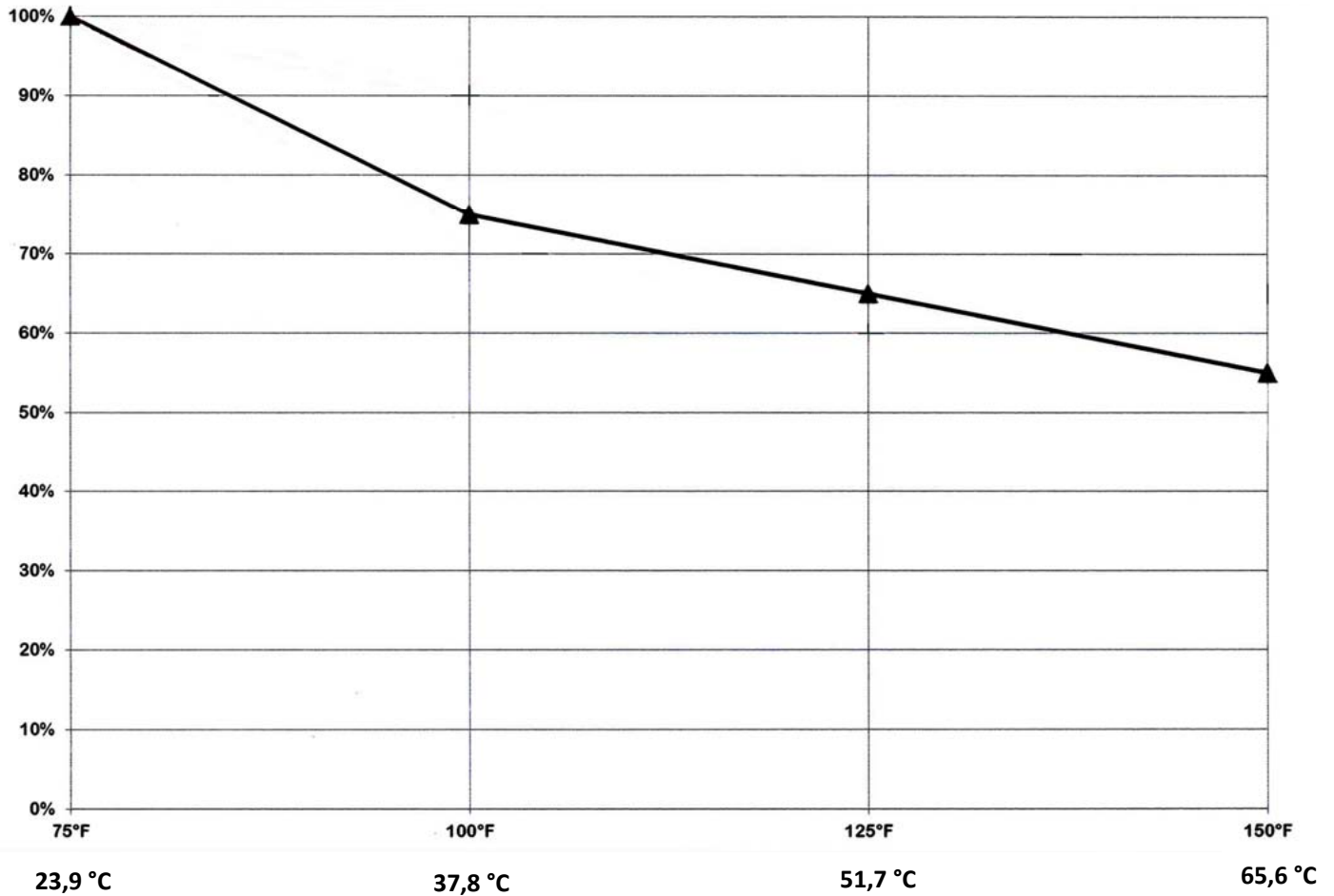
Druck-/Temperatur-Diagramm der Spiralschläuche aus Nylon (PA):
