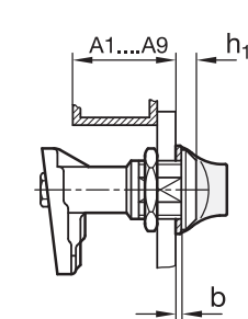
Türverriegelung GN 119
