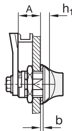
Verriegelungen GN 115
