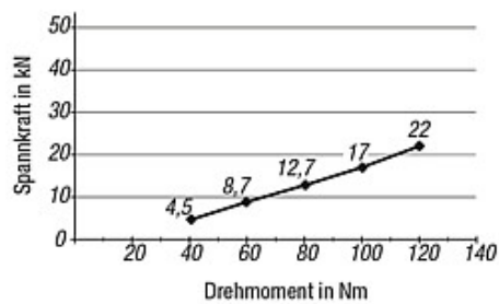
Spannkraft 3-Achs-Spanner
