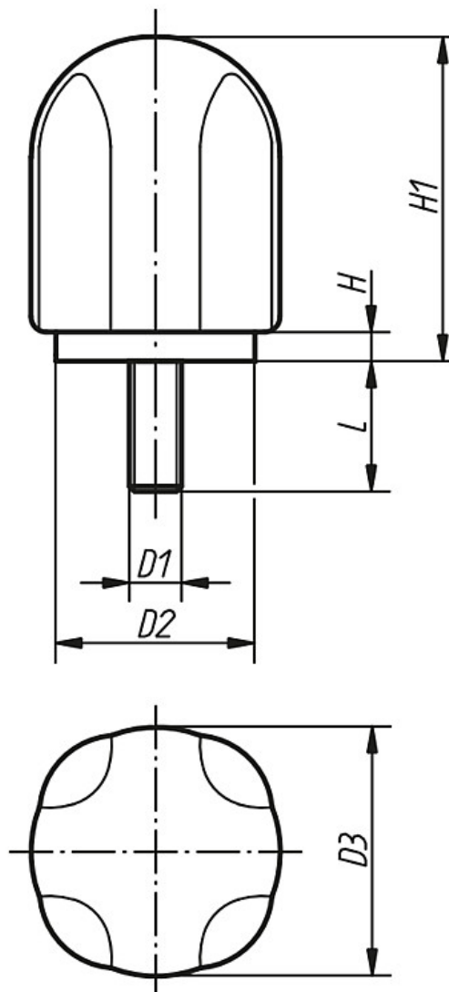
Form L Außengewinde
