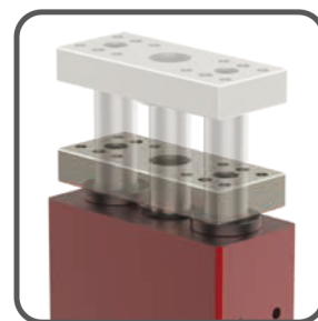
Einstellbarer Hub bis zu 60 mm
