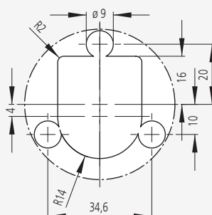
Montageöffnung Mounting cutout
