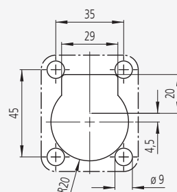
Montageöffnung Mounting cutout
