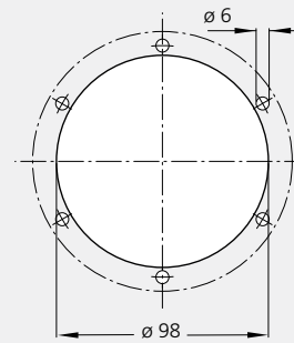
Montageöffnung Mounting cutout
