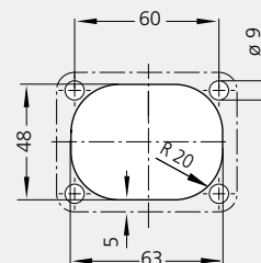
Montageöffnung Mounting cutout
