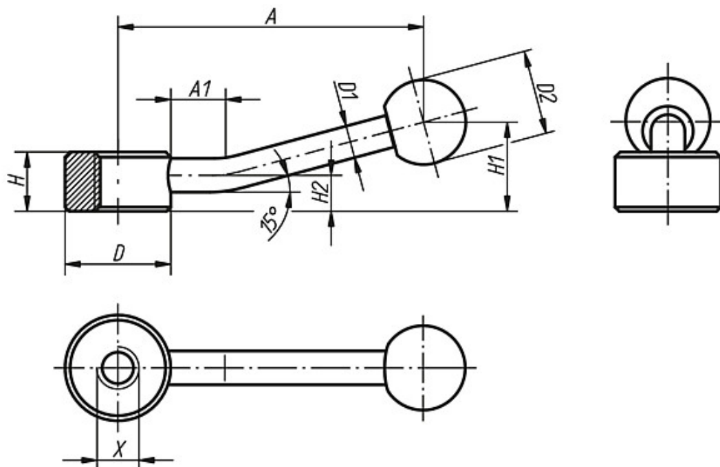
Schaltgriff flach mit Innengewinde
