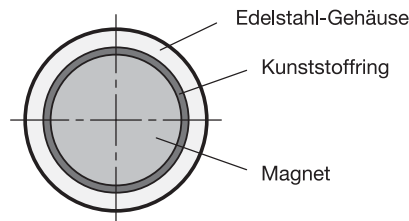
Ansicht auf Haftfläche
