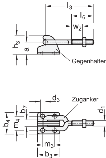
Form TG Zuganker mit Öse
