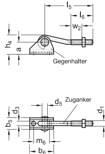
Form TU Zuganker mit Haken
