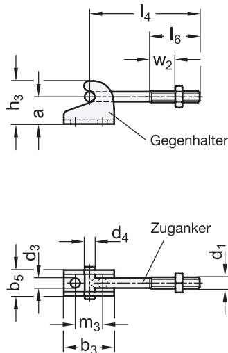
Form TT Zuganker mit T-Stück
