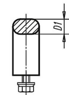
Schnitt A-A
