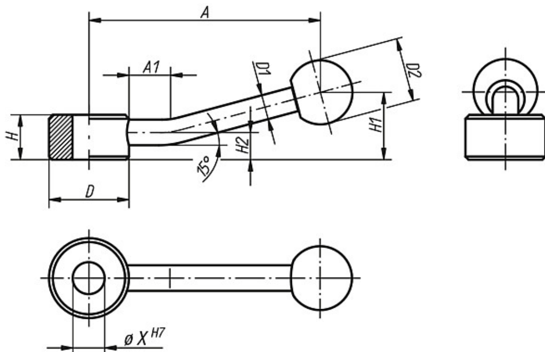
Schaltgriff flach mit Passbohrung
