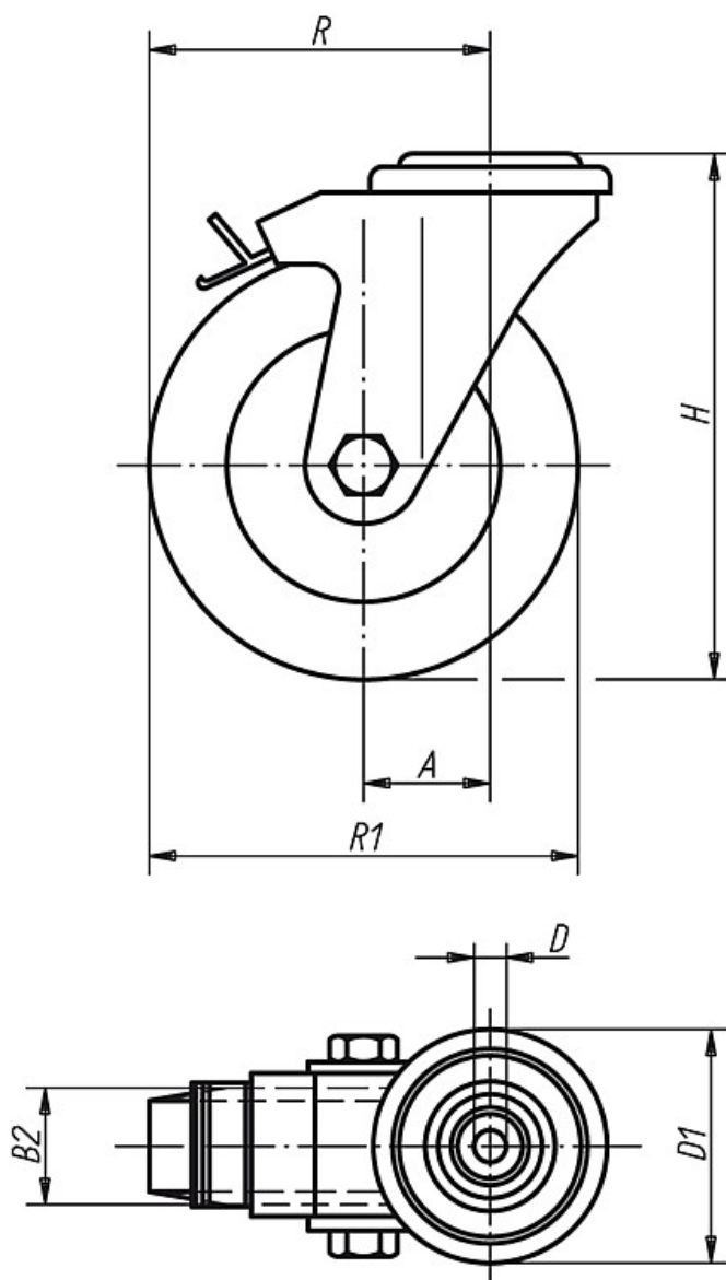
Lenkrolle
