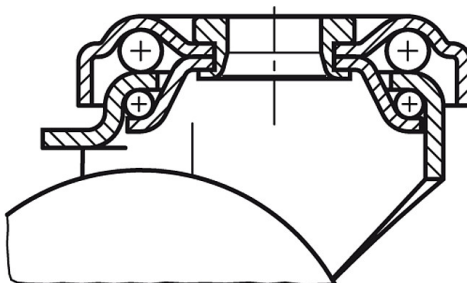
Drehkranzlagerung:
