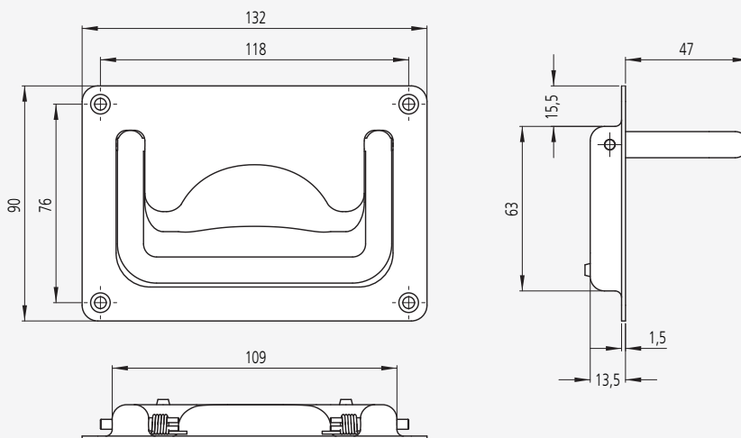
Typ EE-07
